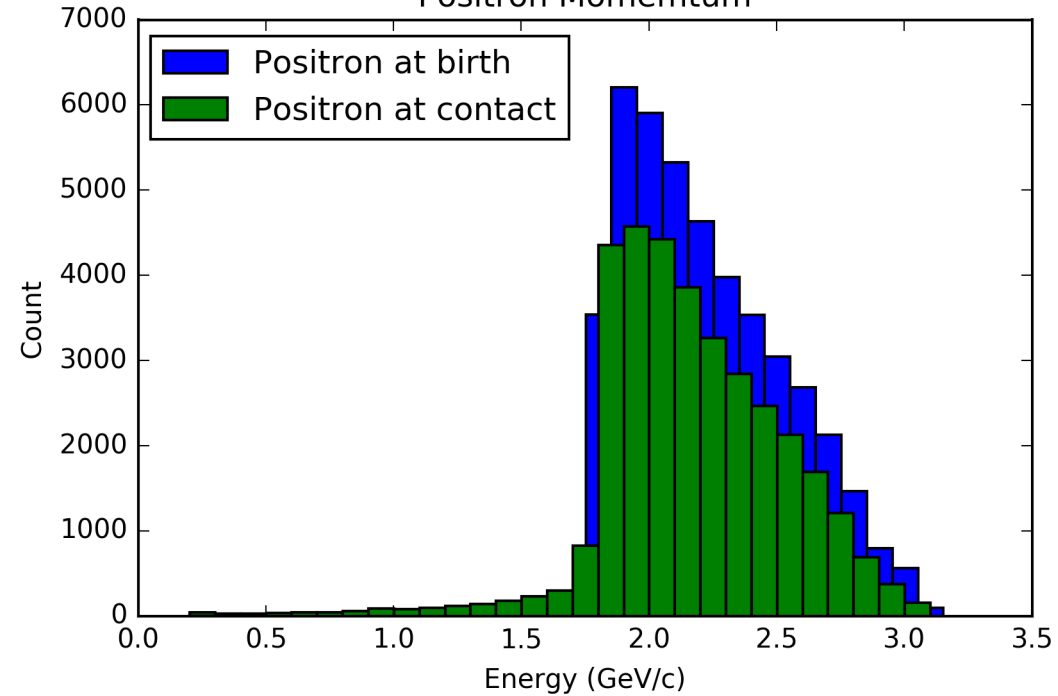
Positron Momentum
